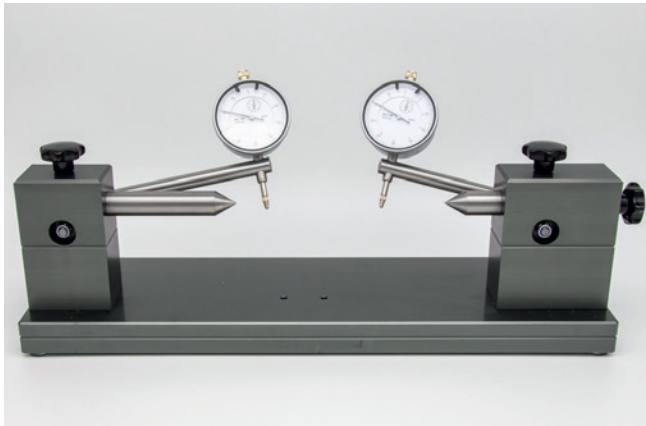
KURBELWELLENRICHTGERÄT 2 (ohne Laufbock) CRANKSHAFT MEASURING SYSTEM 2 (without guidance)
