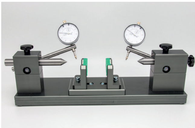
KURBELWELLENRICHTGERÄT 3 (mit Laufbock) CRANKSHAFT MEASURING SYSTEM 3 (with guidance)
